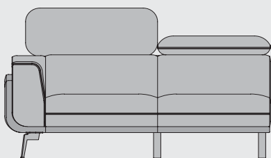
2,5-Sitzer Armlehne links / rechts B166 x T106 x H81/100 cm Art: 33104 (l) / art: 33103 (r)
