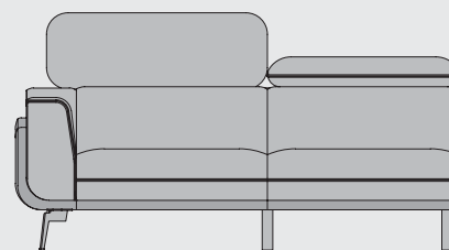
3-Sitzer Armlehne links / rechts B186 x T106 x H81/100 cm Art: 33106 (l) / art: 33105 (r)
