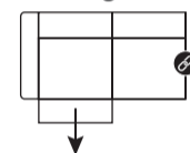
art. nr. 57614/57615 179x77/98x105/158 cm 3-places flex avec accoudoir, 1 x réglable électrique droit/gauche
