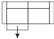
art. nr. 56355/56358 198x106x98/159cm 3,5-Sitzer flex 1 x elektrisch verstellbar rechts/links
