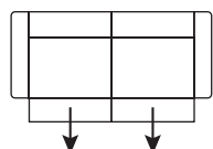
art. nr. 57611 224x77/98x105/158 cm 3,5-places flex 2 x réglable électrique
