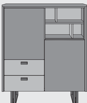
Schrank B120 x T45 x H142,5 cm | 2 Türen + 2 Laden + 4 Nischen art: 29285
