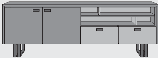
Sideboard B225 x T45 x H77,5 cm | 2 Türen + 2 Laden + 4 Nischen art: 29281
